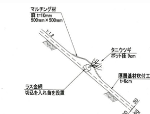
図-9-②苗木設置吹きつけ工概要図
