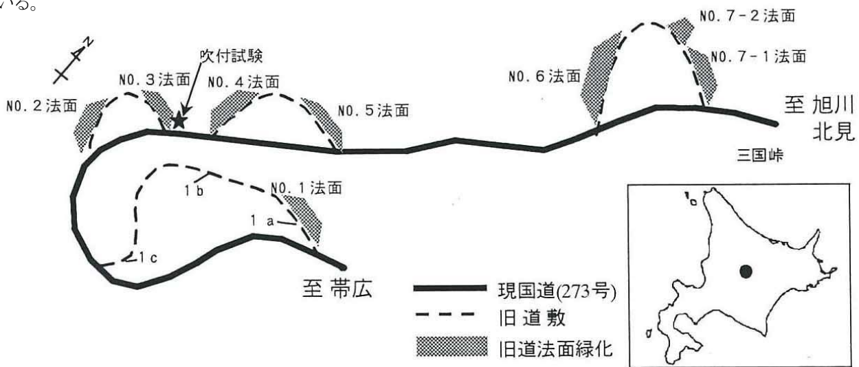
図-8 調査箇所の平面図
