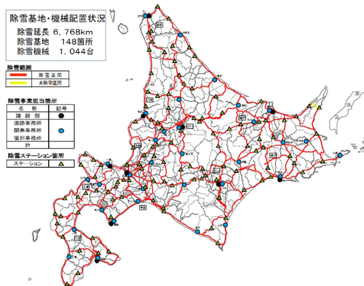
図-1 H29除雪概要図及び機械配置
