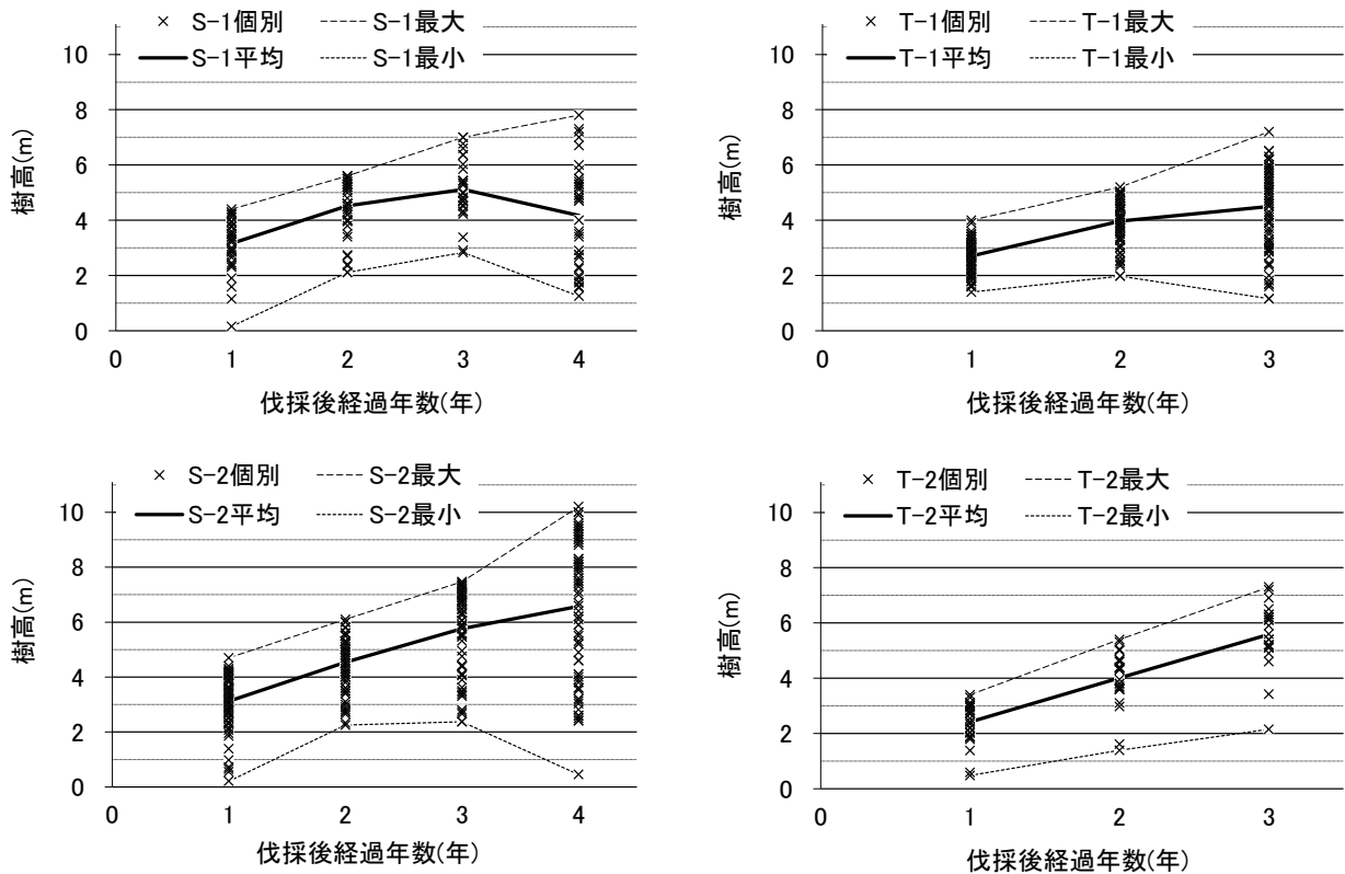
図-3 樹高の推移 (左:猿別川, 右:徳富川)
