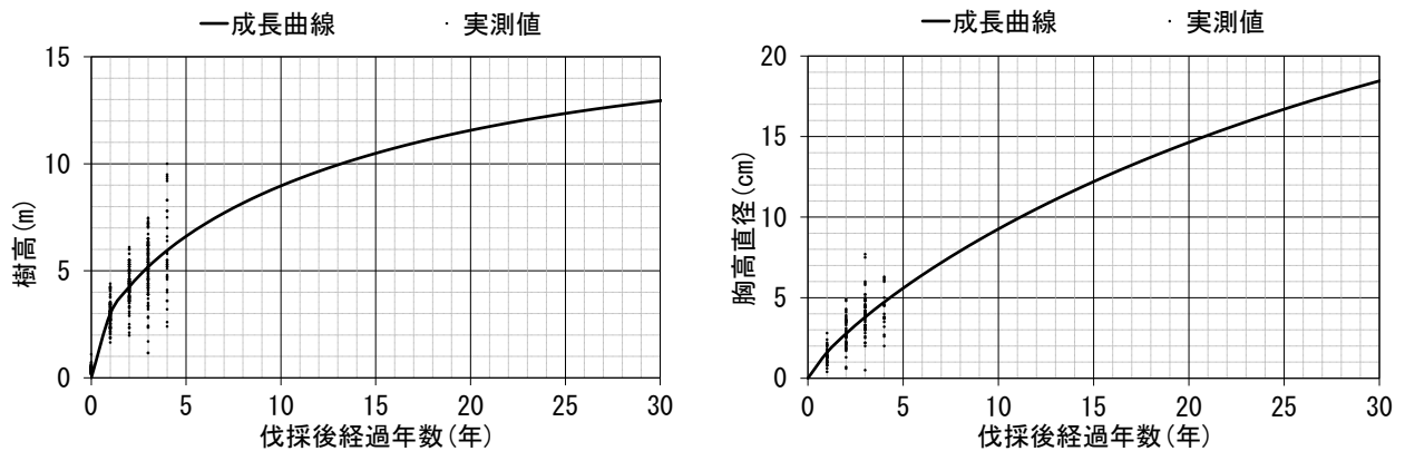
図-6 ヤナギ類河道内樹木の伐採後成長曲線の推定結果 (左:樹高, 右:胸高直径)
