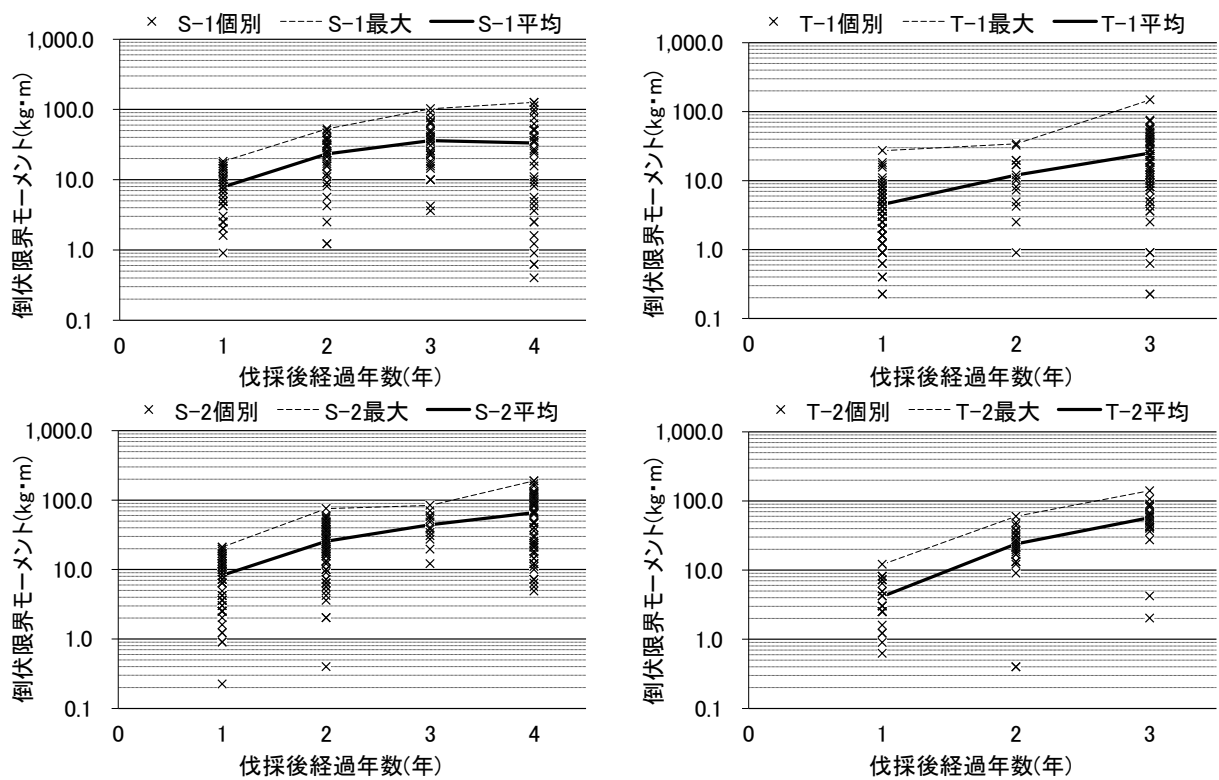
図-5 倒伏限界モーメントの推移 (左:猿別川, 右:徳富川)
