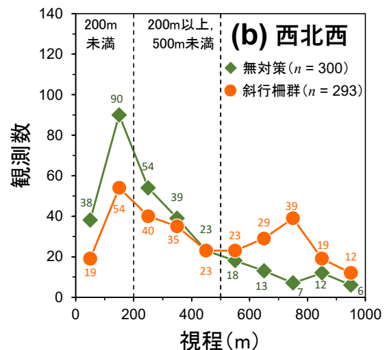
図7 開口部対策の有無による視程別観測数の比較（直交風）
