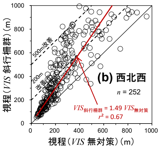
図-4 開口部対策の有無による視程の比較(直交風) (a)西風と(b)西北西風。赤:回帰式、 r^2 :決定係数、 n :データ数。
