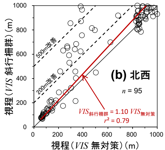
図-5 開口部対策の有無による視程の比較(斜風) (a)西南西風と(b)北西風。その他は図-4に同じ。
