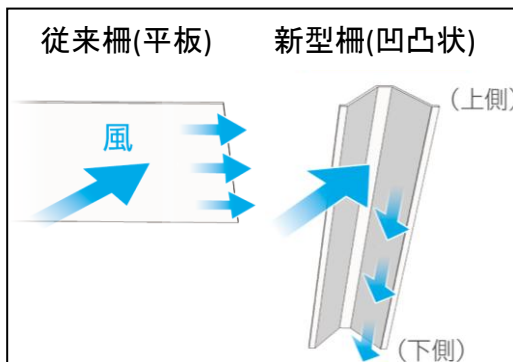
図-3 防雪板の効果イメージ
