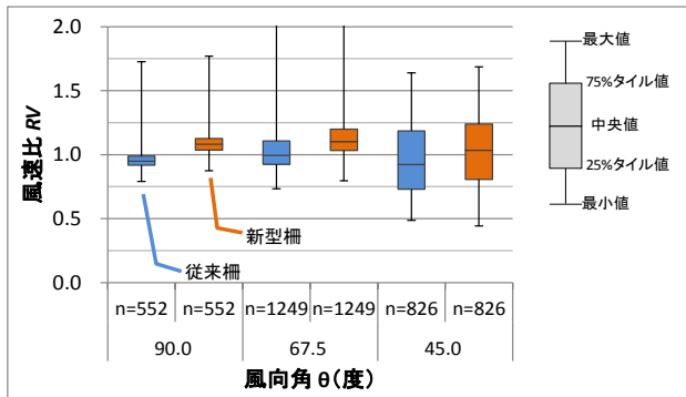
図-6 \theta と RV の関係 ( h=0.5\text{m} )
