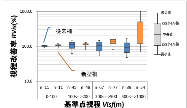
図-10 Vis_f と RV_{is} の関係 ( \theta=45^\circ )
