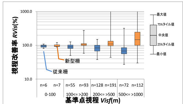
図-9 Vis_f と RV_{is} の関係 ( \theta=67.5^\circ )
