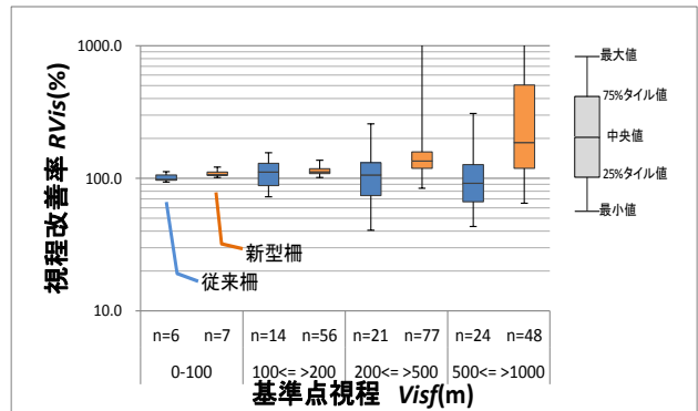
図-8 Vis_f と RV_{is} の関係 ( \theta=90^\circ )
