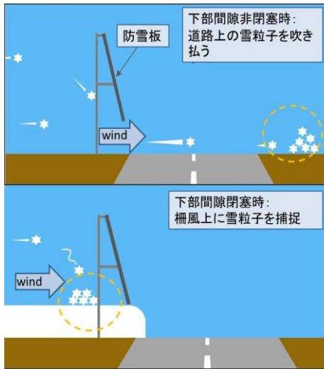
図-2 新型柵の下部間隙閉塞前後における防雪効果イメージ
