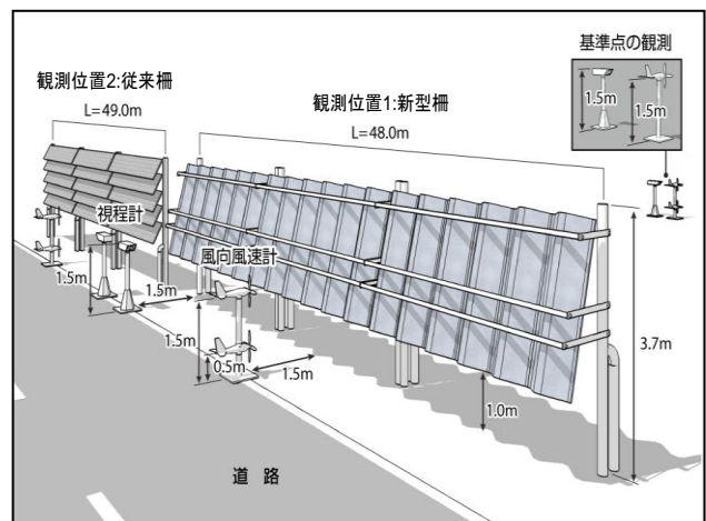
図-5 観測サイトの概要
