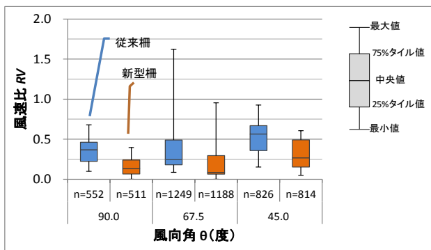
図-7 \theta と RV の関係 ( h=1.5\text{m} )
