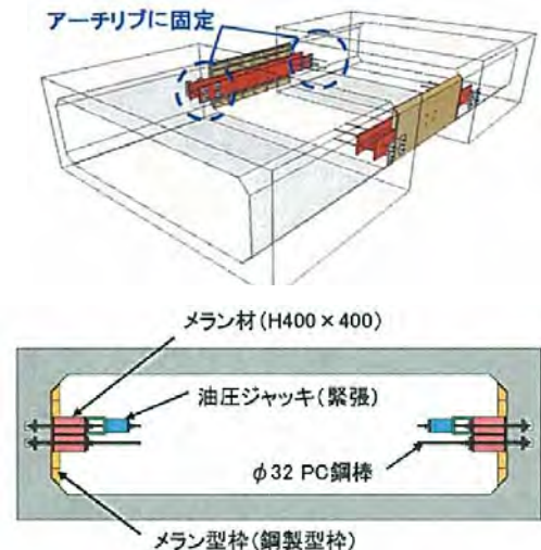
図-5 新メラン工法によるアーチ閉合
