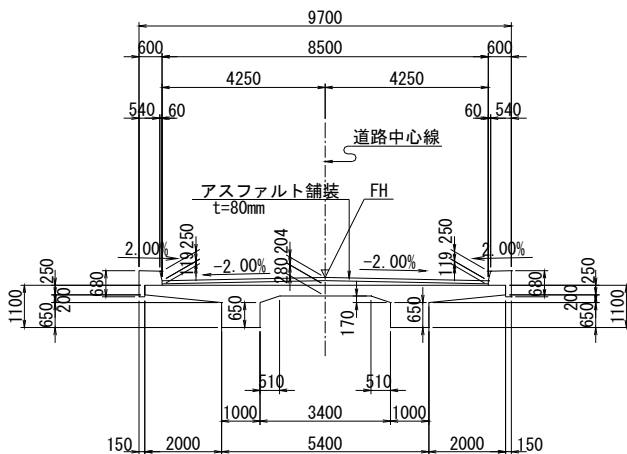
図-6 補剛桁標準断面図
