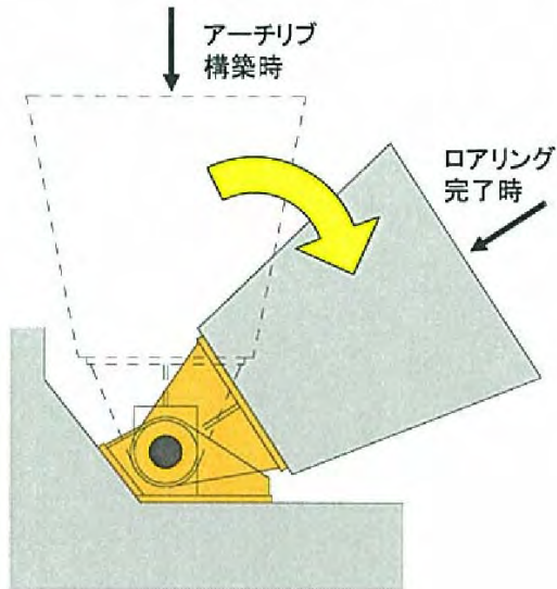
図-4 SM式ロアリング支承
