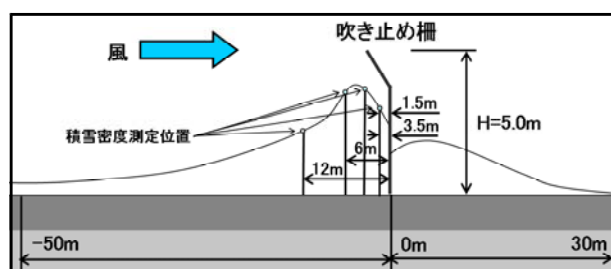
図－2 吹きだまり測定範囲と積雪密度測定位置
