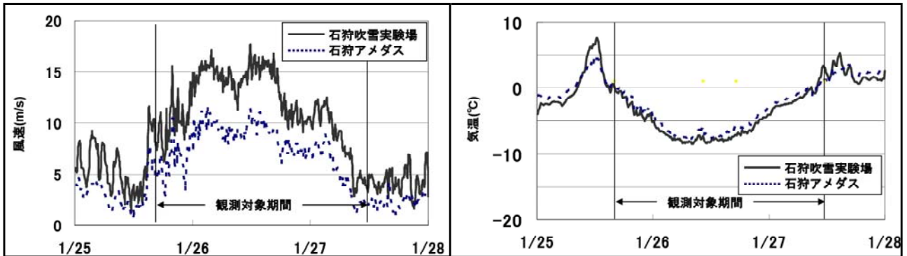
図-5 1月の吹雪時の風速と気温
