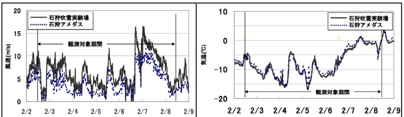
図-6 2月の吹雪時の風速と気温
