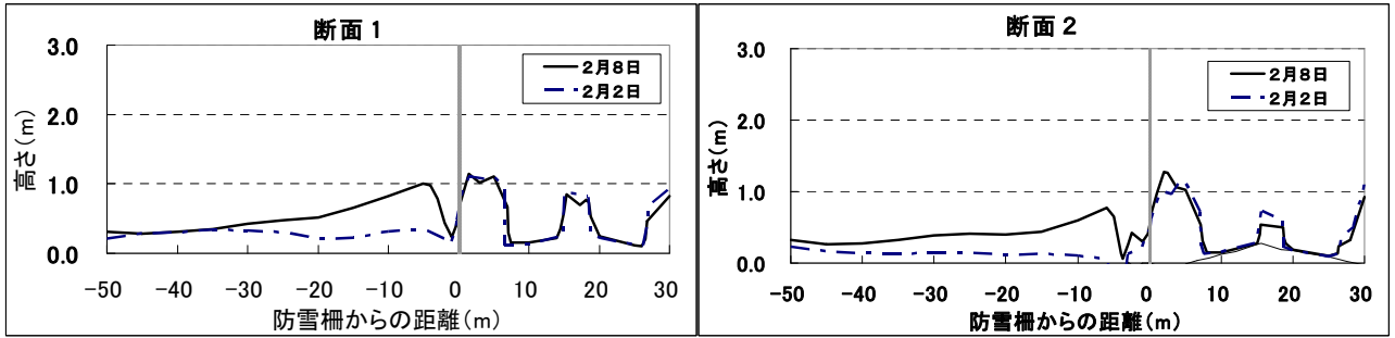
図－4 2月の吹雪時の吹きだまり状況
