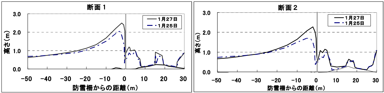
図－3 1月の吹雪時の吹きだまり状況
