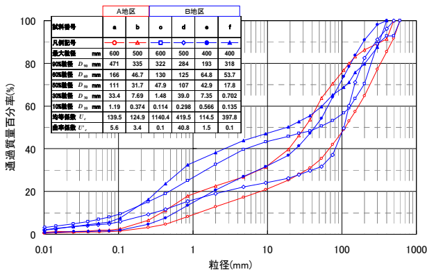
図-3 H18 粒度試験結果 (全量)
