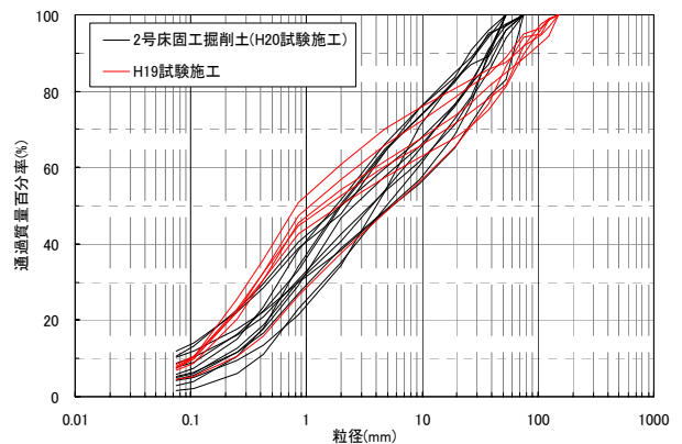
図-4 H19年度およびH20年度の母材粒度
