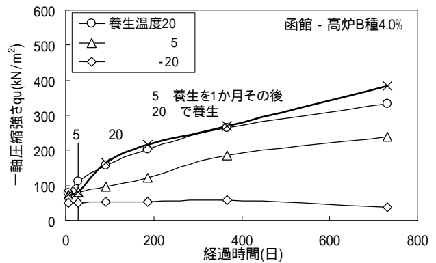
(a) 5、20で養生したときの軸圧縮強さの変化
