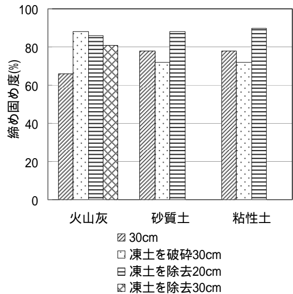
図-7 夏期土工と冬期土工の盛土の締固め度
