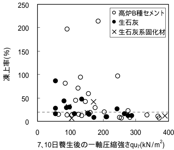
図-6 一軸圧縮強さと凍上率
