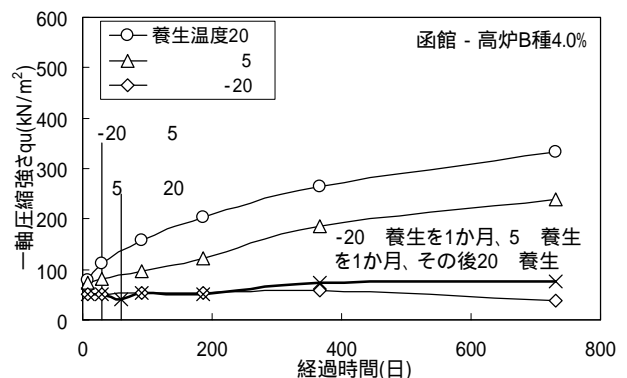
(c) はじめに-20で養生したときの軸圧縮強さの変化
