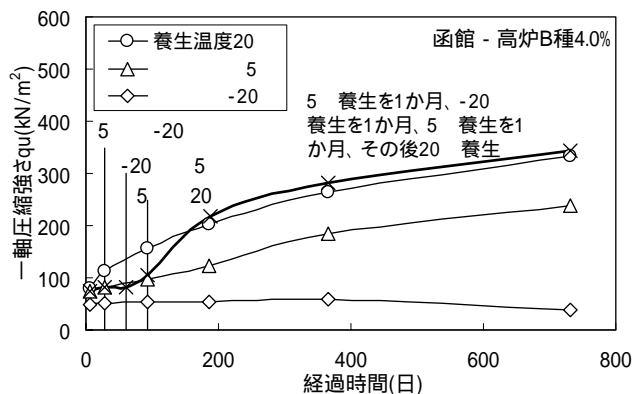
(b) 5、-20、20で養生したときの軸圧縮強さの変化
