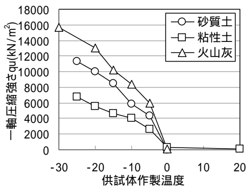
図-1 供試体作製温度と強度
