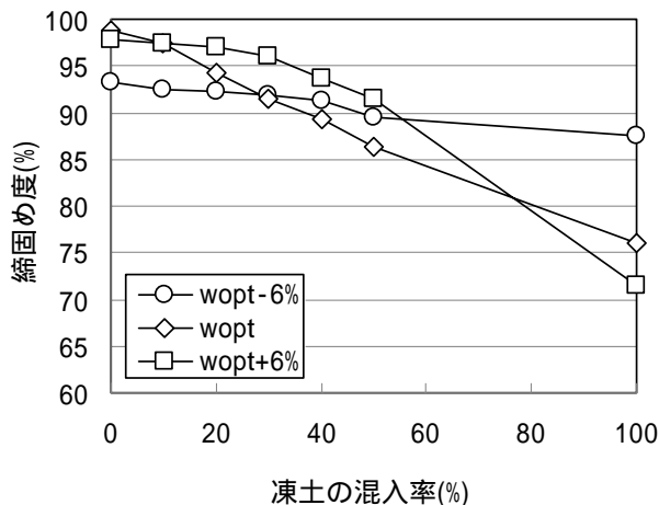
図-3 含水比の違いと凍土の混入率と締め固め度
