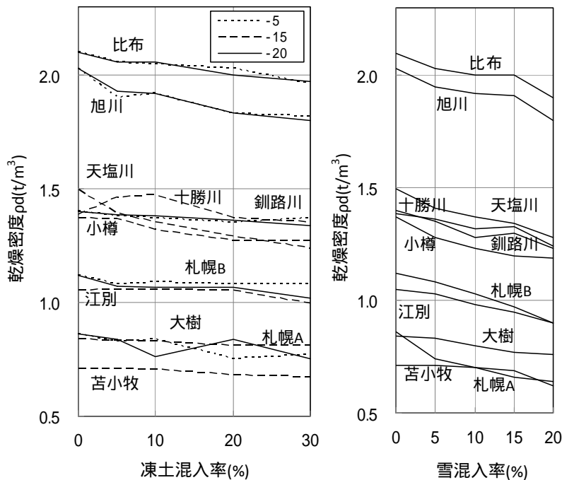
図-2 凍土または雪混合による締め固め密度への影響
