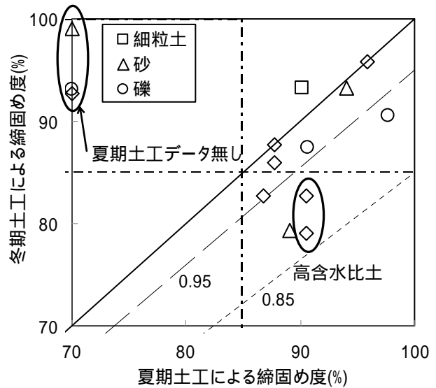
図-7 夏期土工と冬期土工の盛土の締固め度
