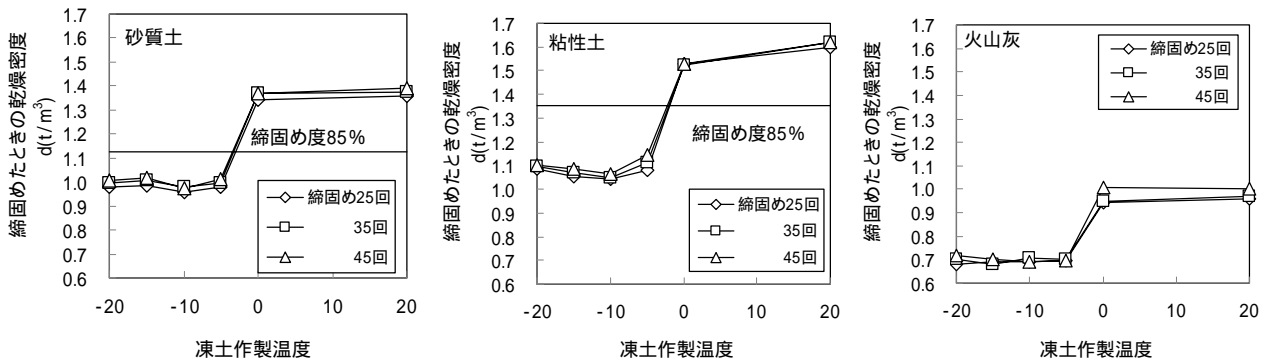
図-4 施工時の気温と締固め密度の関係
