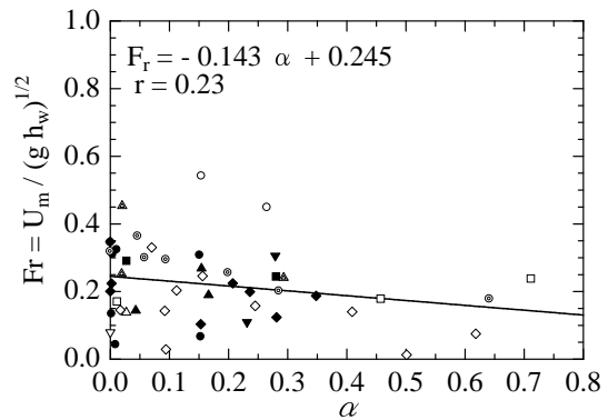
図-17 係数 \alpha と F_r
