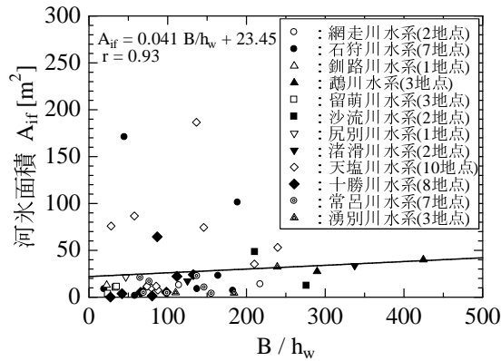
図-8 川幅水深比 B/h_w と河水面積 A_{if}
