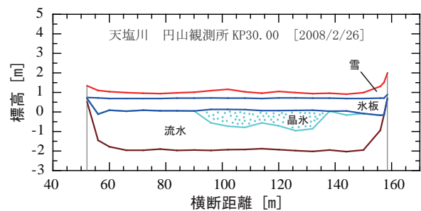
図-1 河川結氷時の横断面図の一例
