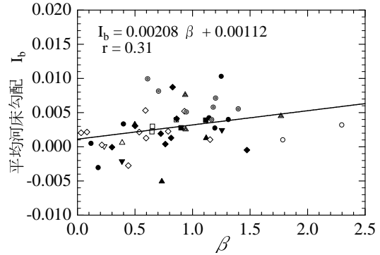
図-12 係数 \beta と平均河床勾配
