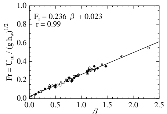
図-18 係数 \beta と F_r
