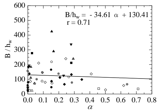
図-13 係数 \alpha と川幅水深比 B/h_w
