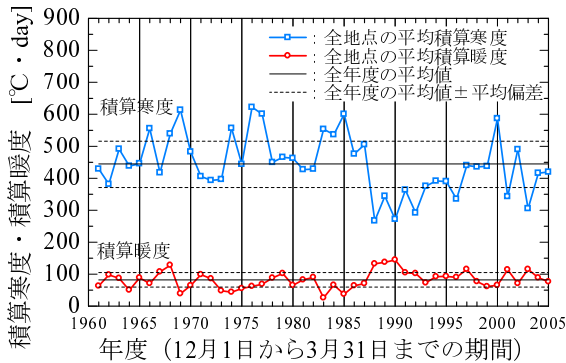
図-4 1961年度から2005年度における積算寒度および積算暖度
