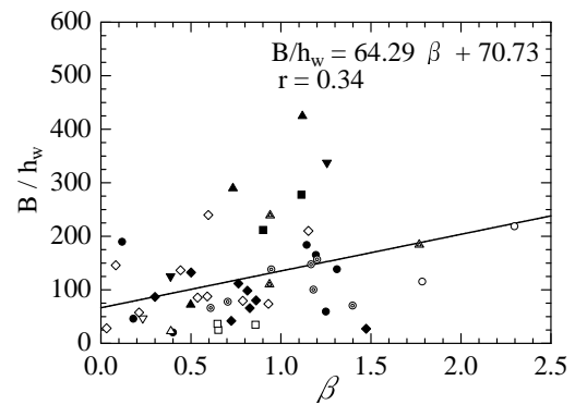
図-14 係数 \beta と川幅水深比 B/h_w
