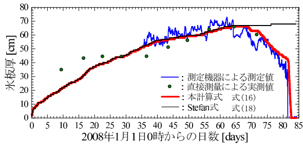
図-6 氷板厚の測定値と計算値
