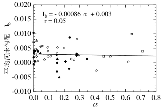
図-11 係数 \alpha と平均河床勾配
