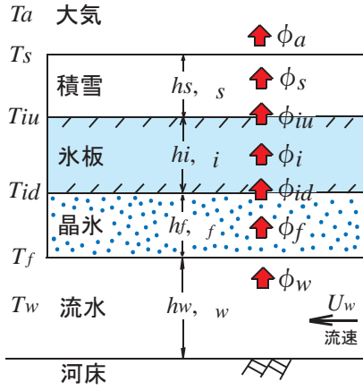
図-5 結氷河川における熱収支の概要図
