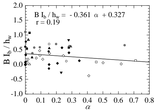
図-15 係数 \alpha と BI_b/h_w
