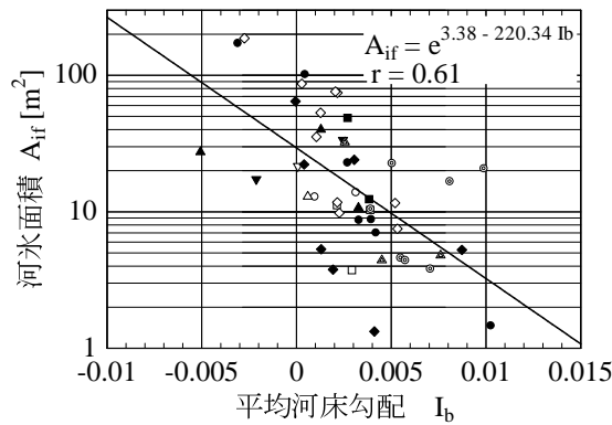
図-9 平均河床高 I_b と河水面積 A_{if}
