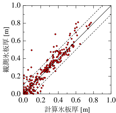
図-7 氷板厚の計算値と観測値
