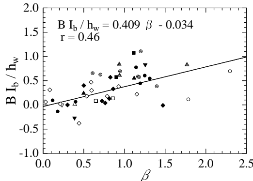
図-16 係数 \beta と BI_b/h_w
