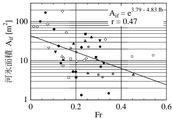
図-10 フルード数 Fr と河水面積 A_{if}
