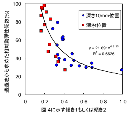
図-5 表面走査法のグラフから求める直線の傾きと透過法から求めた相対動弾性係数の関係 (深さ10mm位置と深さ t 位置)
