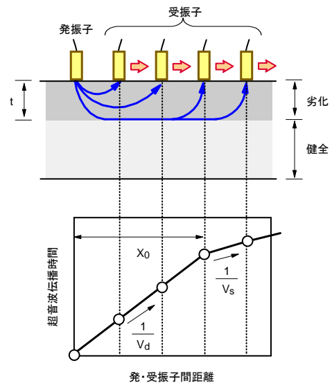
図-1 表面走査法
