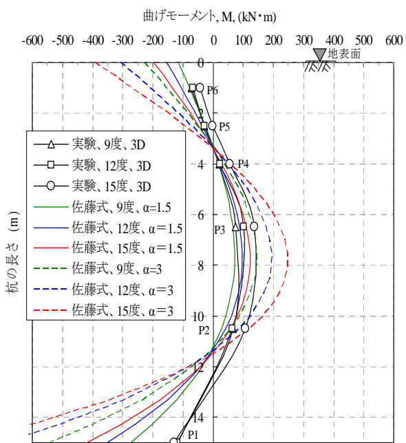
図-6 斜杭 \theta の違いの杭曲げモーメント
