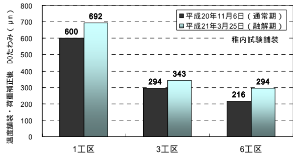
図-11 稚内試験舗装における通常期と融解期の D0 たわみ
