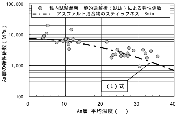
図-6 逆解析によるAs層の弾性係数と4点曲げ疲労試験から得た曲げスティフネス
