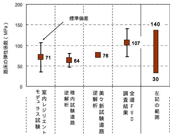
図-8 路床土の弾性係数の範囲
